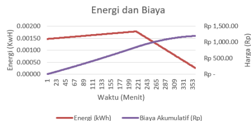
Gambar 7. Hasil Energi dan Biaya Selama Pengisian Berlangsung
