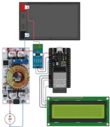
Gambar 4. Rangkaian Pengujian Sensor ACS712 30A
