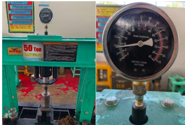
Gambar 1. Proses pencetakan dan tekanan yang diberikan pada cetakan
