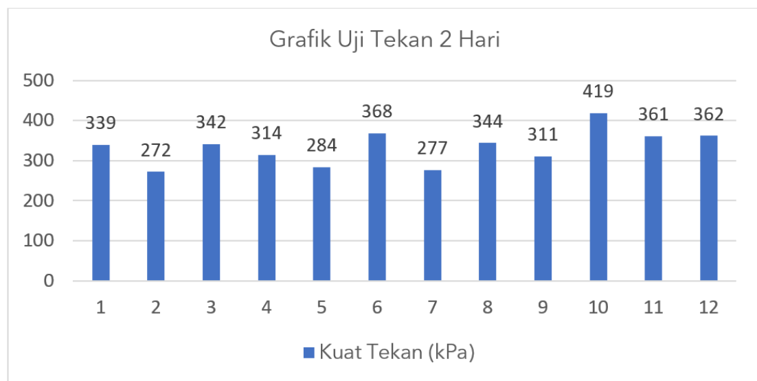
Gambar 3. Grafik Pengujian Tekan Penjemuran 2 Hari
