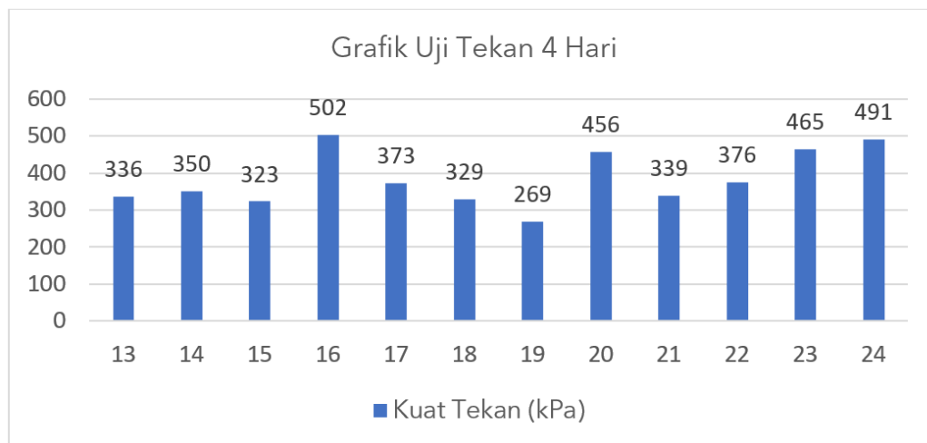
Gambar 4. Grafik Pengujian Tekan Penjemuran 4 Hari
