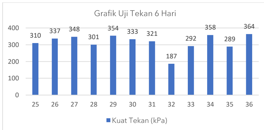
Gambar 5. Grafik Pengujian Tekan Penjemuran 6 Hari
